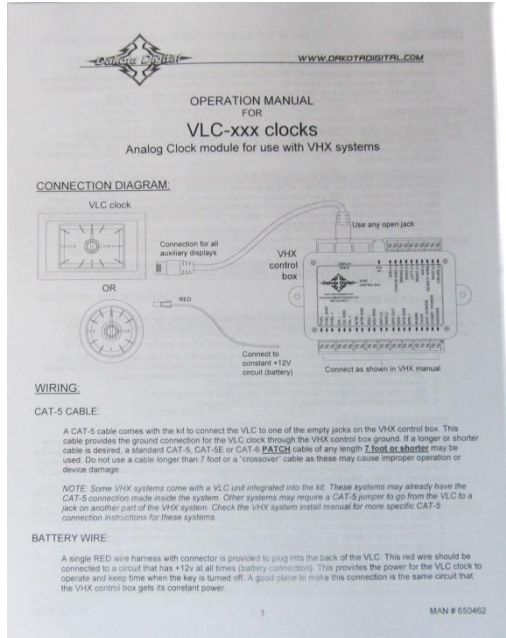
CAT5 Cable
